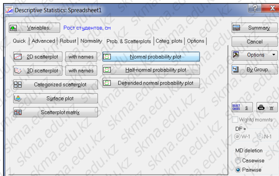
Рисунок 8. Построение нормального вероятностного графика
